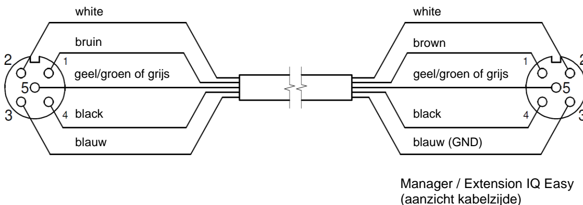
Afbeelding 11: Bedrading Thunder/ ON IQ aan IQ Easy platform
