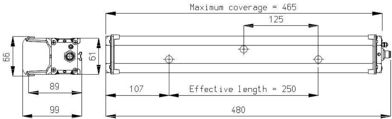
Afbeelding 2: Afmetingen Thunder/ON met 3 emitters
